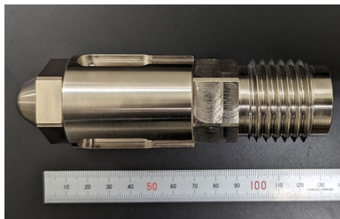
図2 双曲線穴形状を有するダイを挿入した射出ノズル
